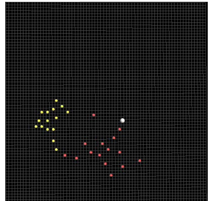
Jäger/Beute Simulation
